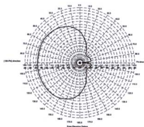
H-Plane Pattern
